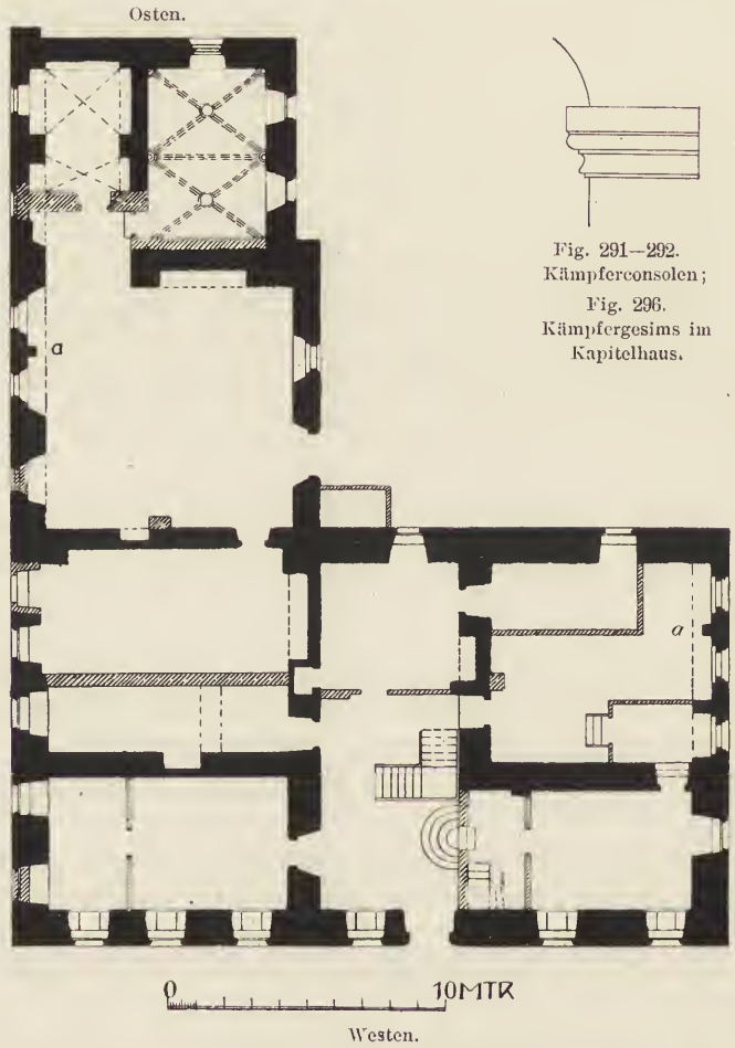
Fig. 293. Grundriss des Abthaus.
